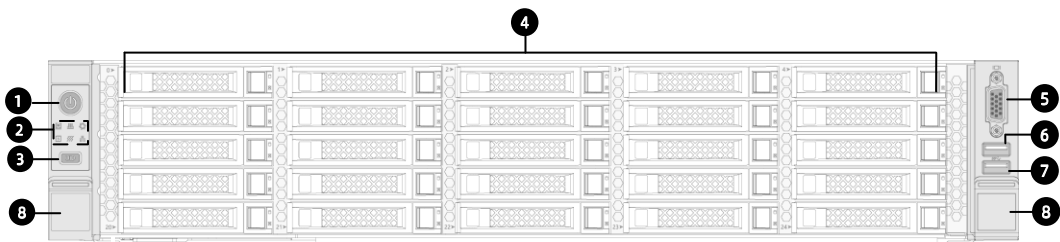
图 5-5 正视图
