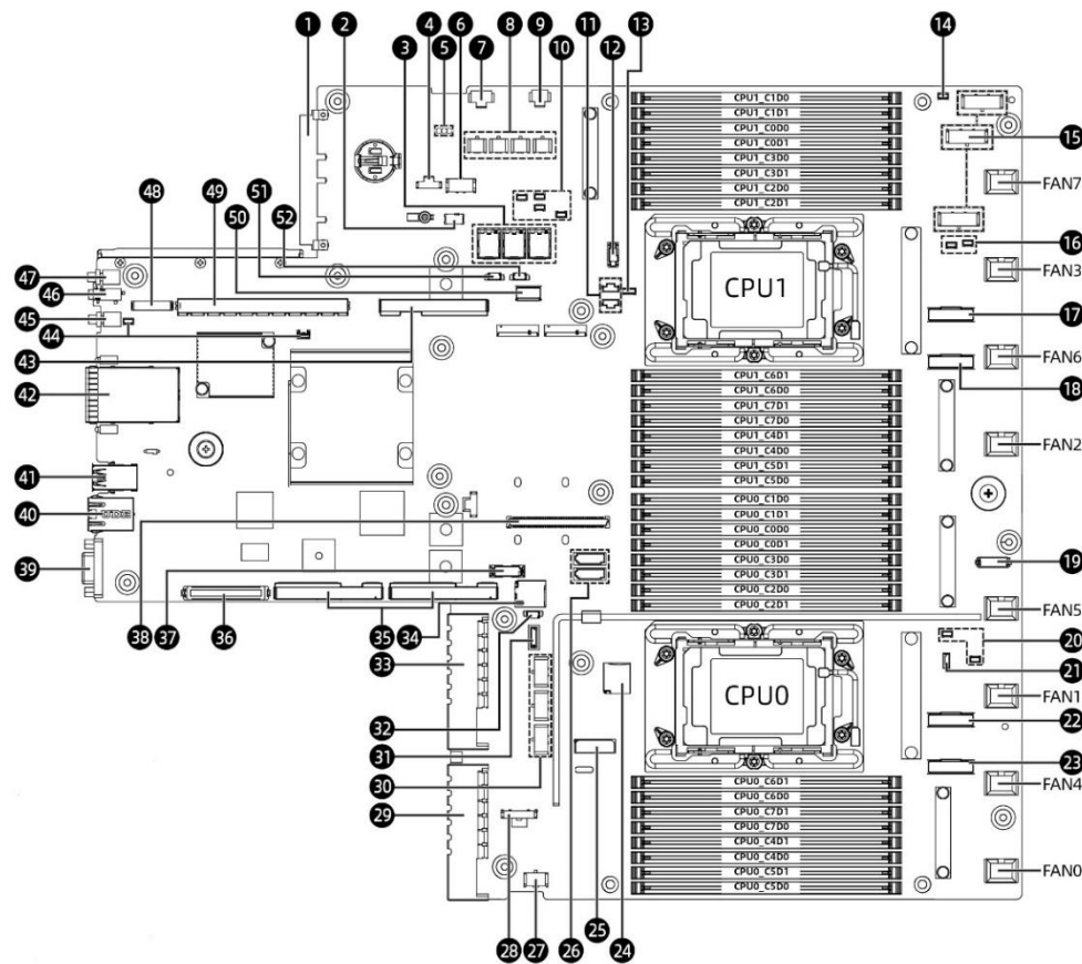
图 5-12 主板图布局
