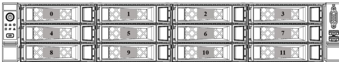
图 7-2 前置(8×2.5")×3
