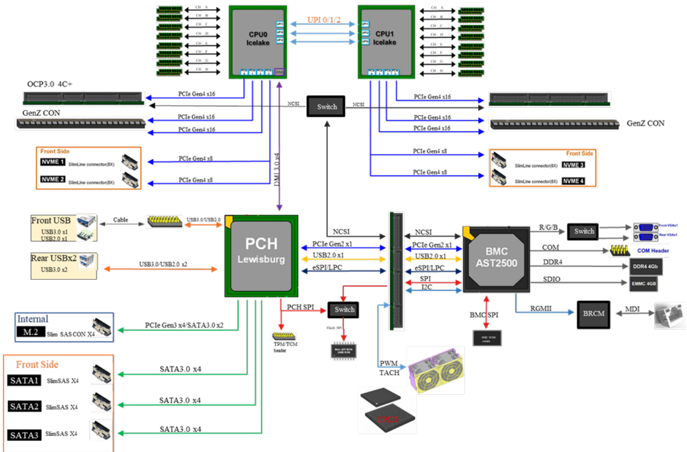
主板布局图
