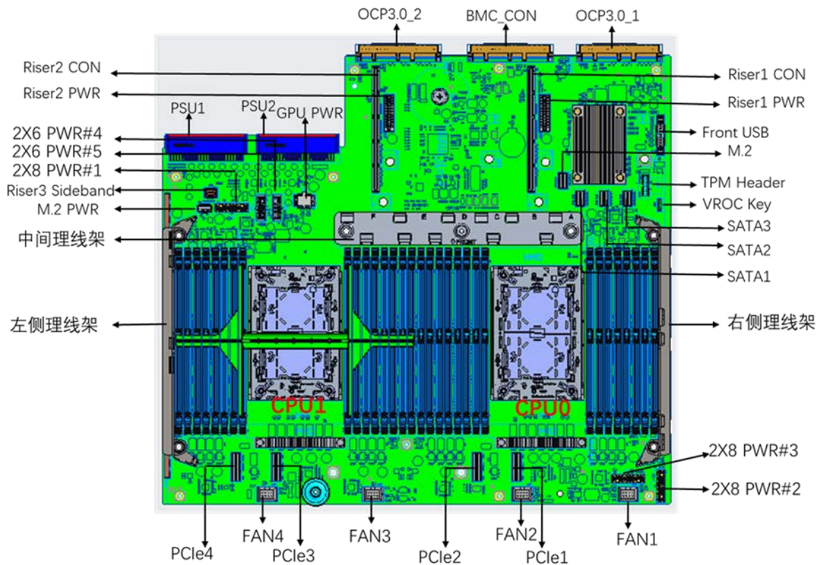
主板布局图
